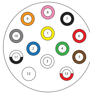
12V 13-polig Steckdose
