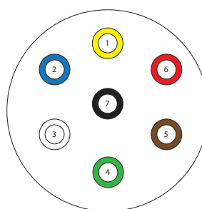
12V 7-polig Steckdose
