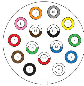
24V 15-polig Stecker
